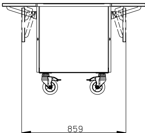
Dessus
